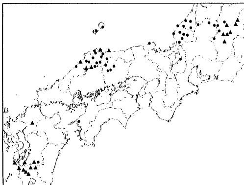
図5 7月18～23日に降水量最大値を更新した観測所 統計期間1979年～2006年で、20年以上の観測値が得られる観測所が対象。▲：24時間降水量および48時間降水量最大値を更新、●：48時間降水量最大値を更新。 +：1時間降水量最大値を更新。
