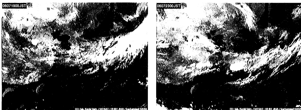
図1 2006年7月18日24時(左)、22日24時(右)の気象衛星赤外画像 高知大学気象情報頁 ( http://weather.is.kochi-u.ac.jp/ ) より引用。
